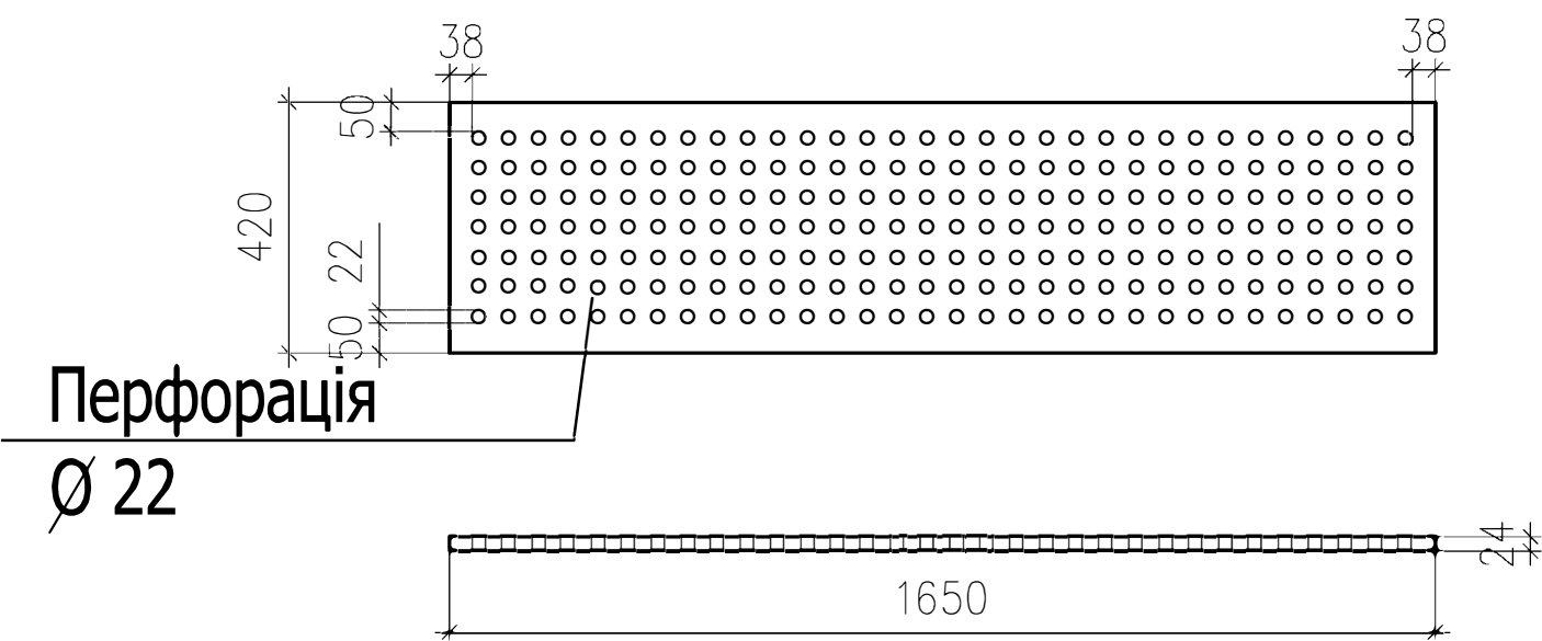
деталь 13 однакова з двох сторін
