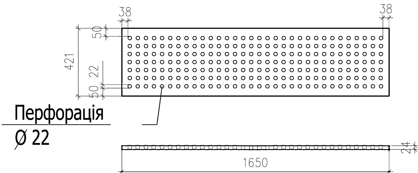
деталь 11 однакова з двох сторін
