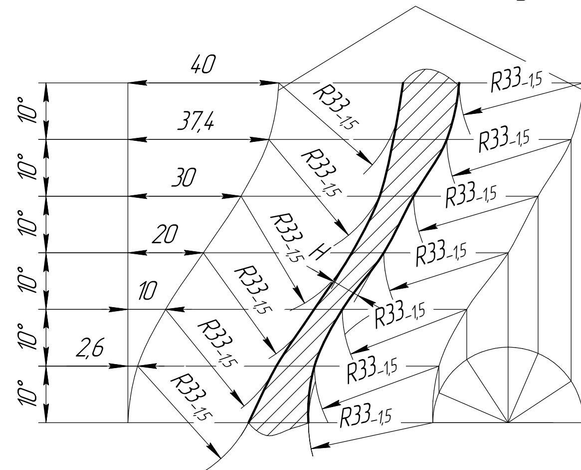
A-AO Профиль гребня Эквивалентные косинусоиды
