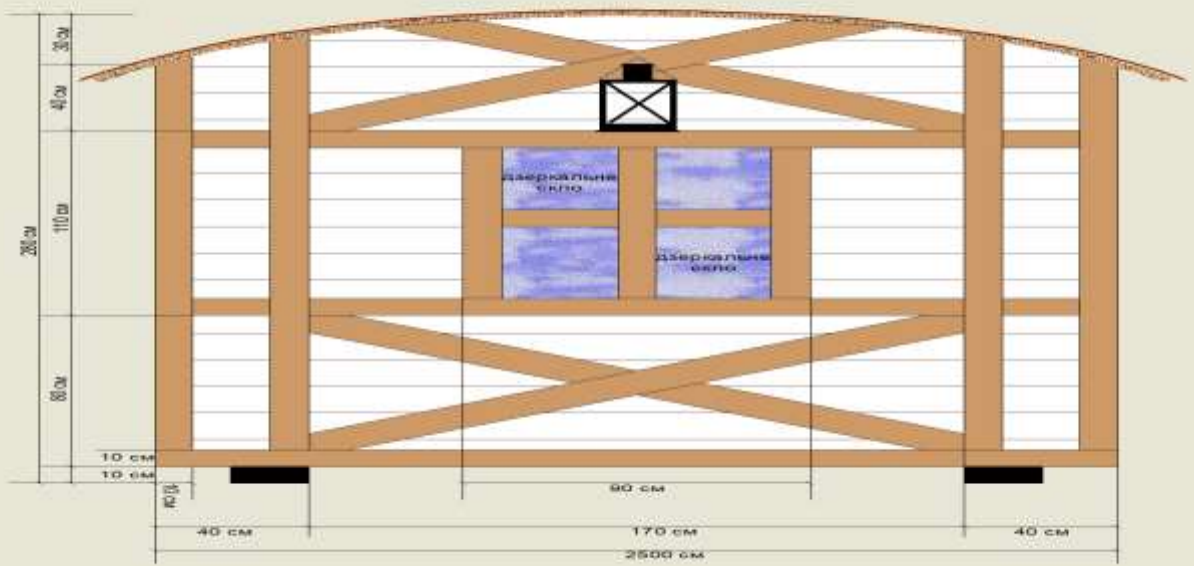
ТОРГВЕЛЬНИЙ КІОСК-ПАРОТЯГ. СХЕМАТИЧНЕ КРЕСЛЕННЯ
