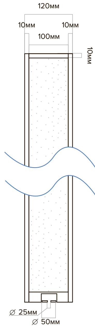
Вид спереду
