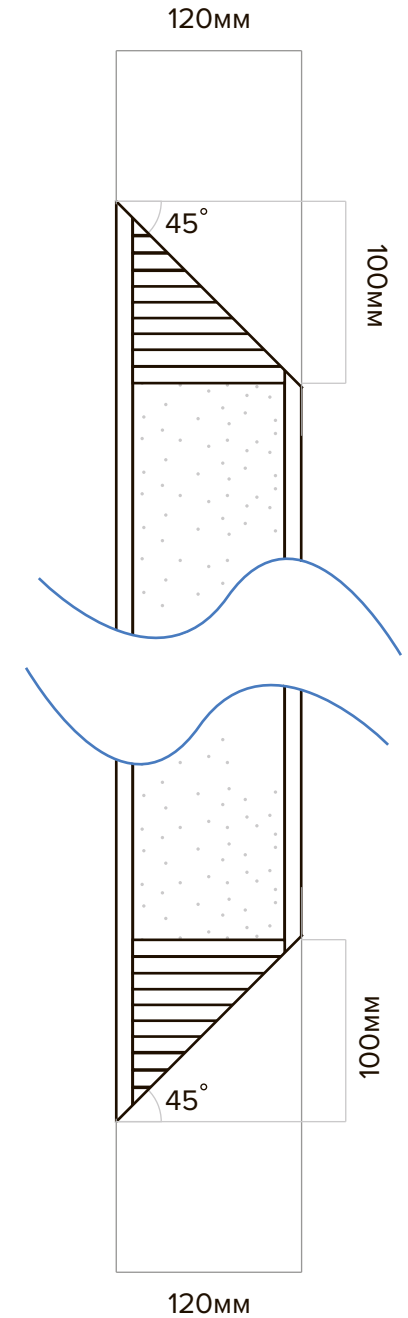
Вид зверху
