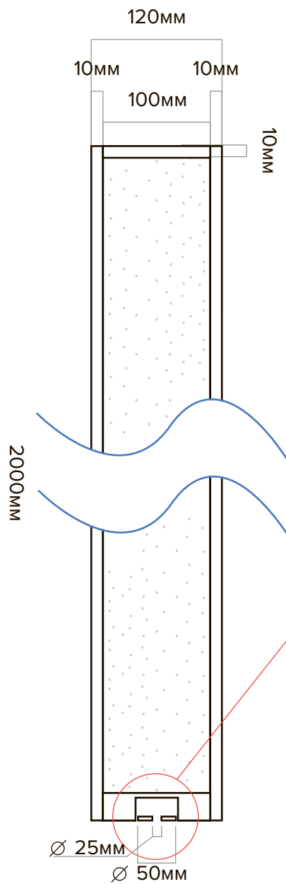
Вид спереду
