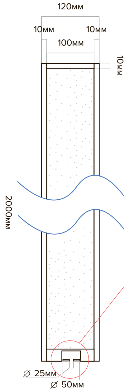
Вид спереду
